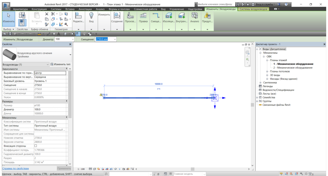
Рисунок 4.39. Окно расчета коэффициента трения в прямом воздуховоде круглого сечения
