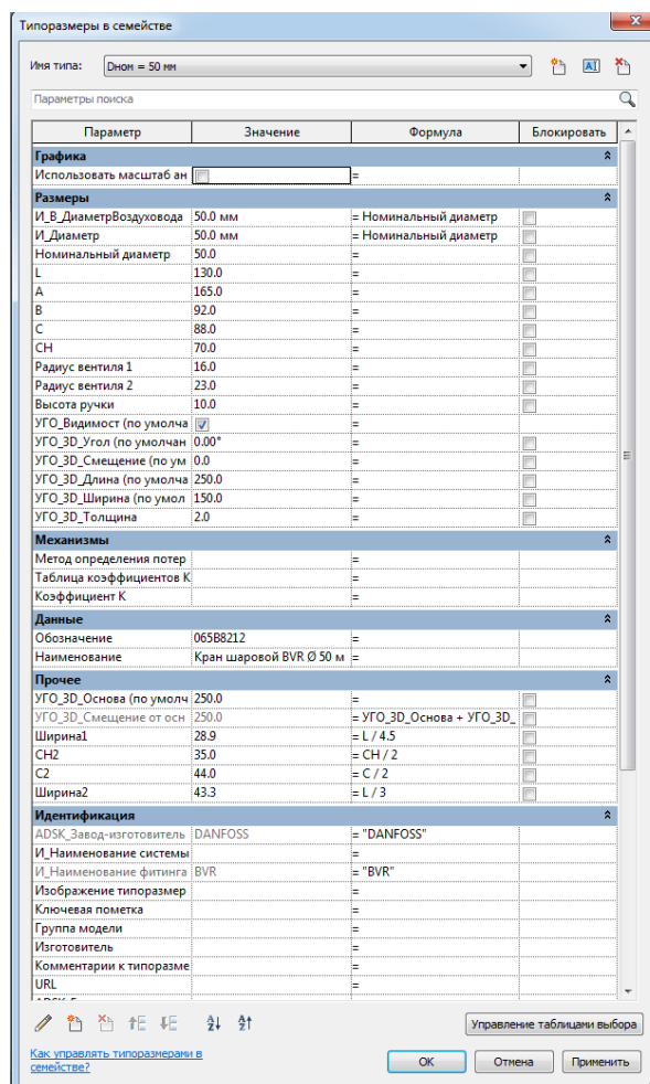
Рисунок 3.20. Окно типоразмеров в семействе элемента
