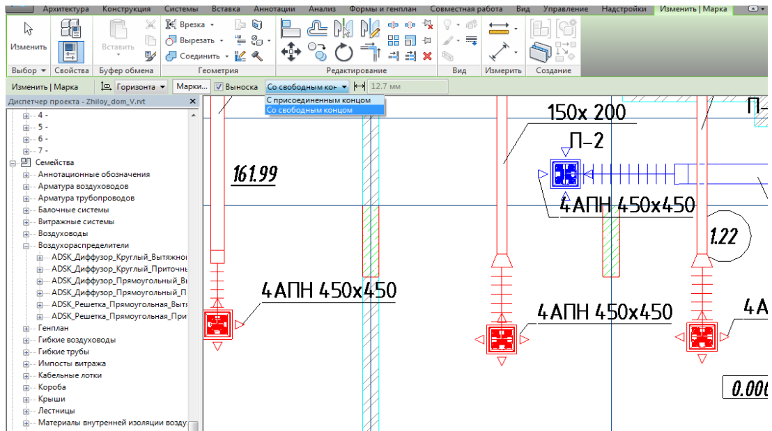
Рисунок 4.15. Маркировка системы, оборудования
