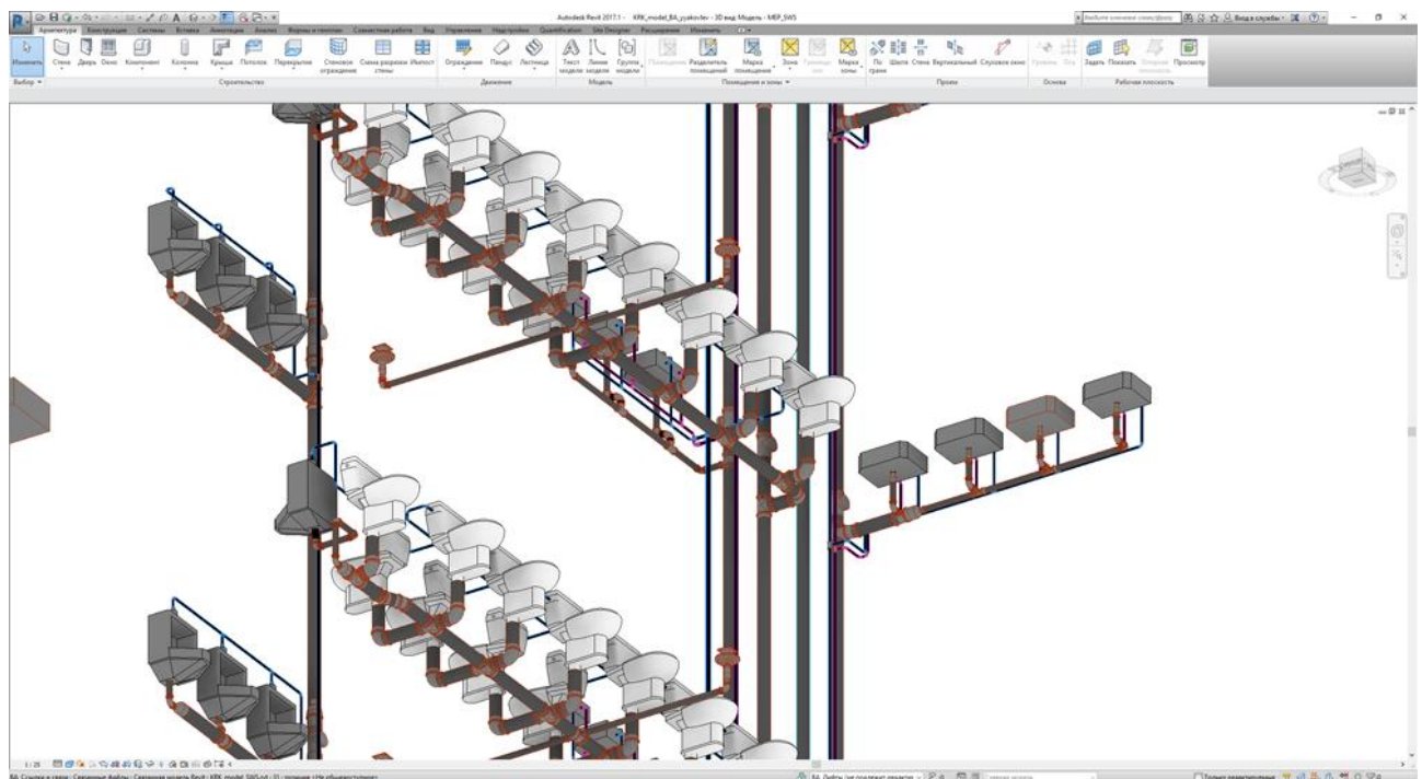
Рисунок 1.4. ВМ-проектирование. Часть системы водоснабжения и отведения стоков здания, представляемая в отдельном окне без строительных конструкций
