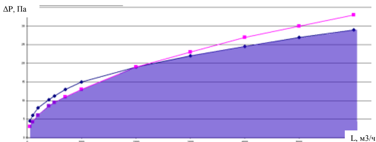
Рисунок 4.41. Определение размеров воздуховодов по трению (—◆—) и скорости (—■—)
