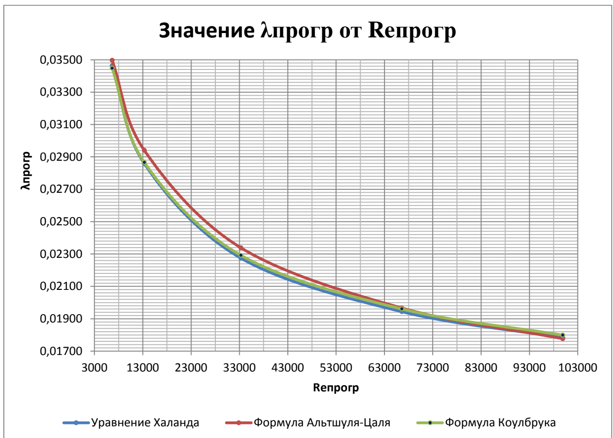
Рисунок 4.40. Результаты расчета зависимости \lambda_{прогр} от Re_{прогр} по формулам Халанда, Коулбрука и Альтшуля.
