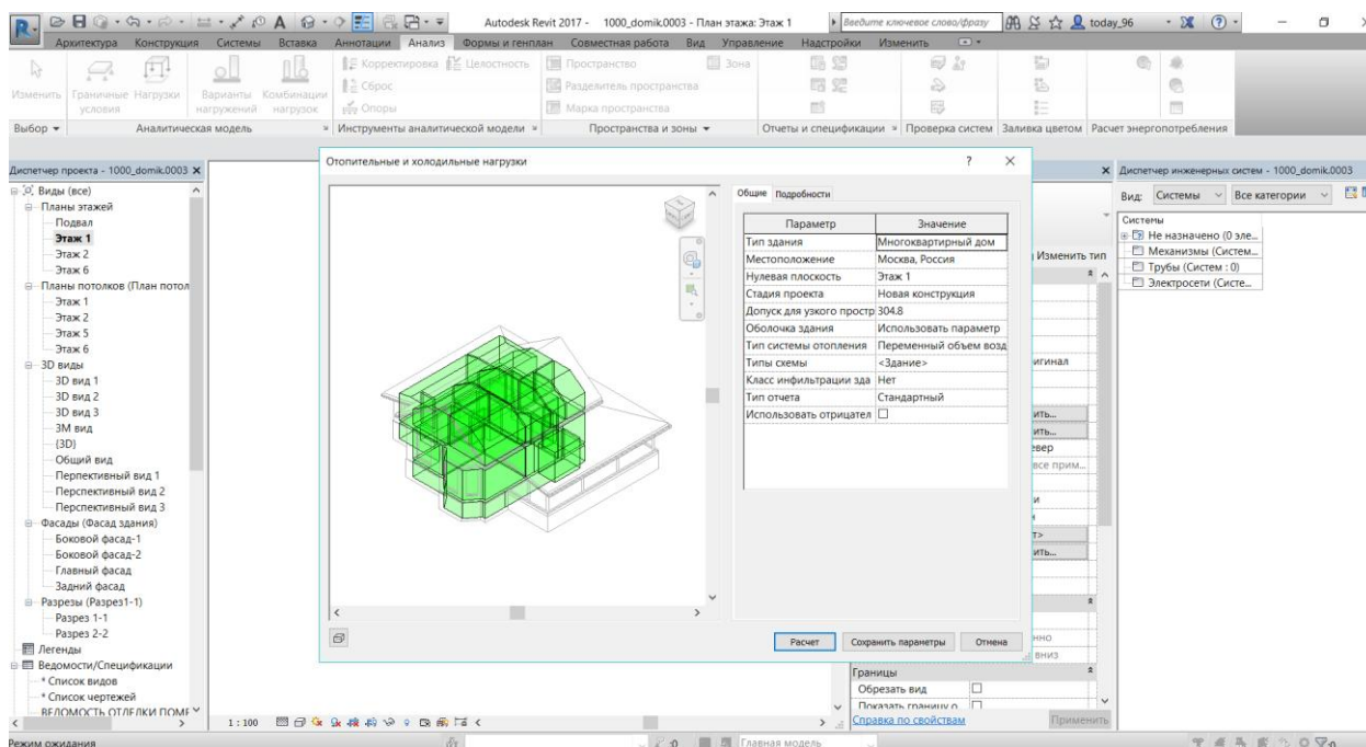
Рисунок 3.77. Диалоговое окно Отопительные и холодильные нагрузки
