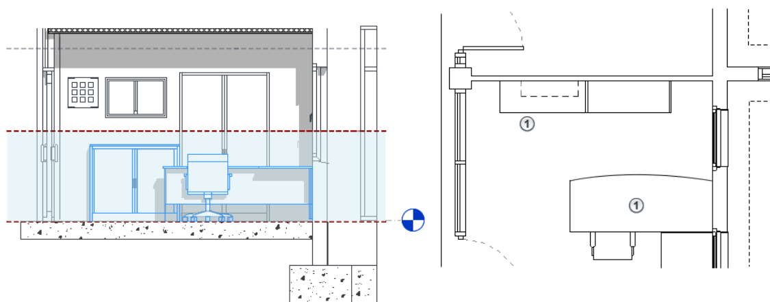
Рисунок 3.47. Пример элементов, находящихся под секущей плоскостью и над нижним пределом секущего диапазона
