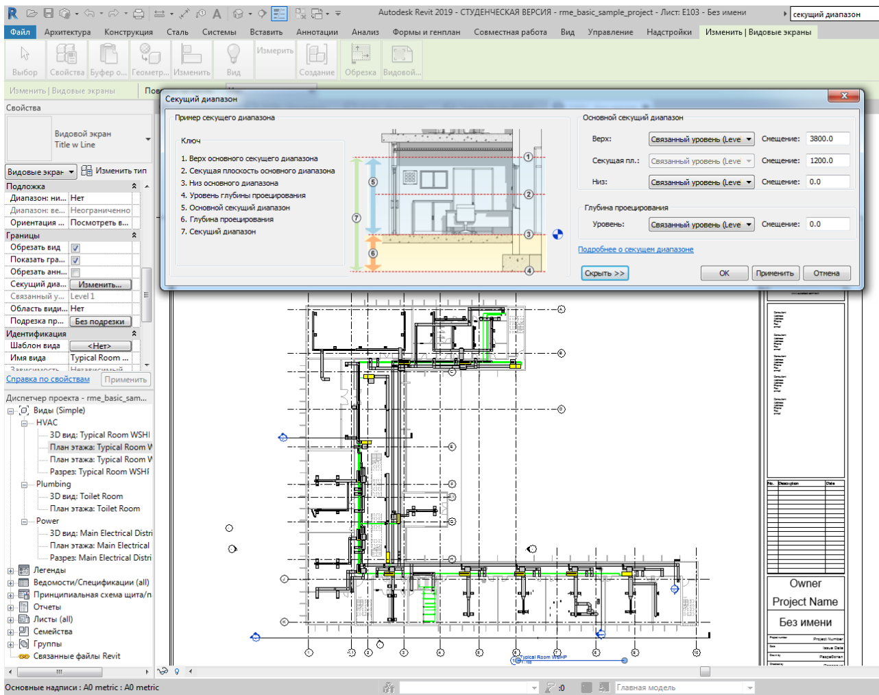
Рисунок 3.42. Диалоговое окно «Секущий диапазон» палитры свойств
