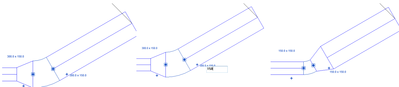
Рисунок 4.30. Изменение размеров фитингов
