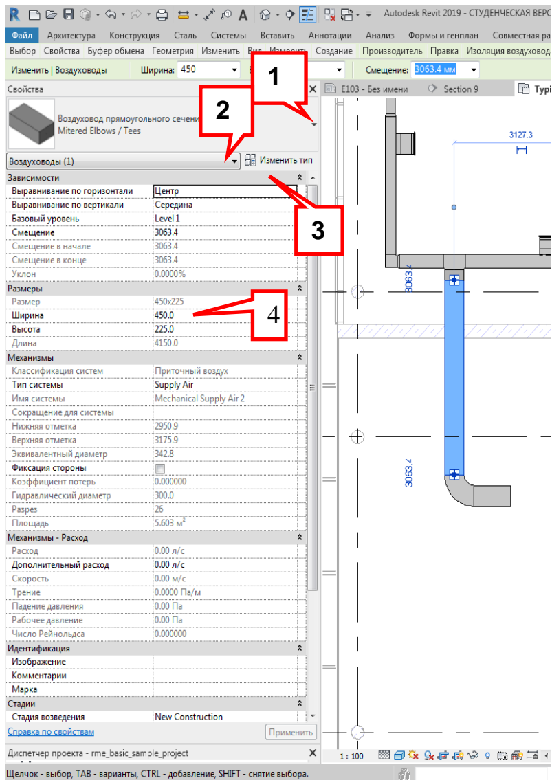
Рисунок 3.6. Палитра свойств для элемента: 1 – выбор типа воздуховода, 2 – фильтр свойств, 3 – кнопка «Изменить тип», 4 – свойства элемента
