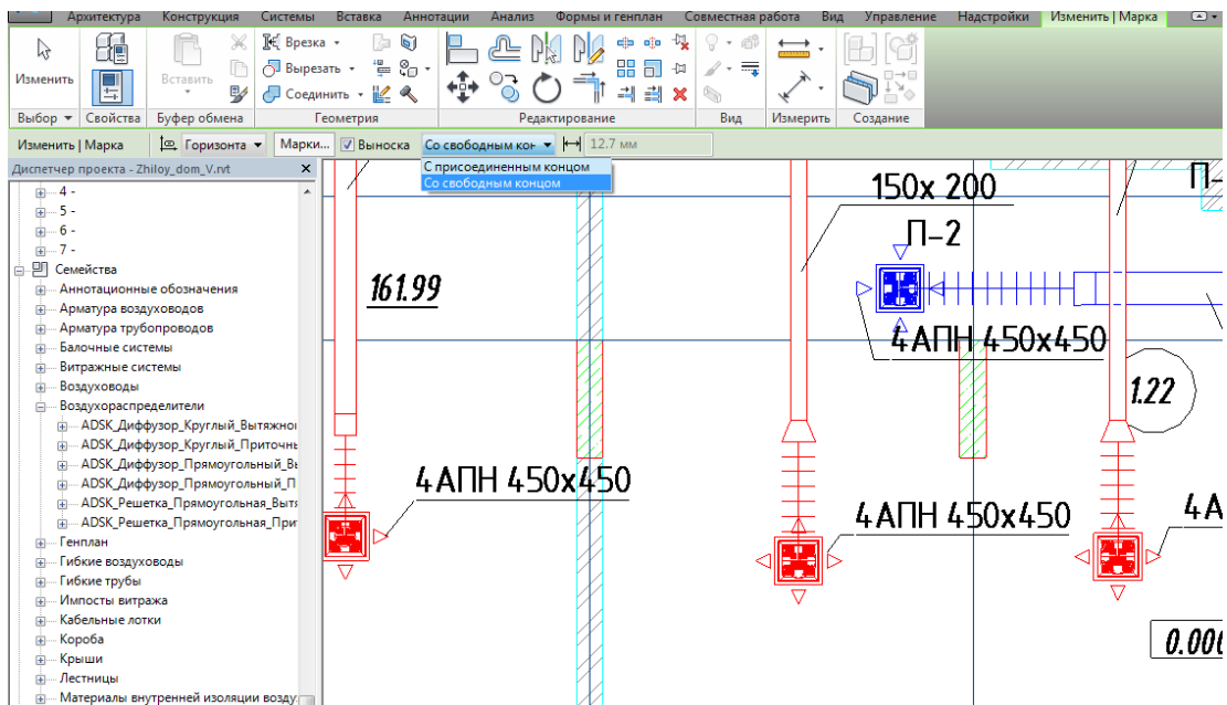
Рисунок 4.38. Маркировка системы, оборудования
