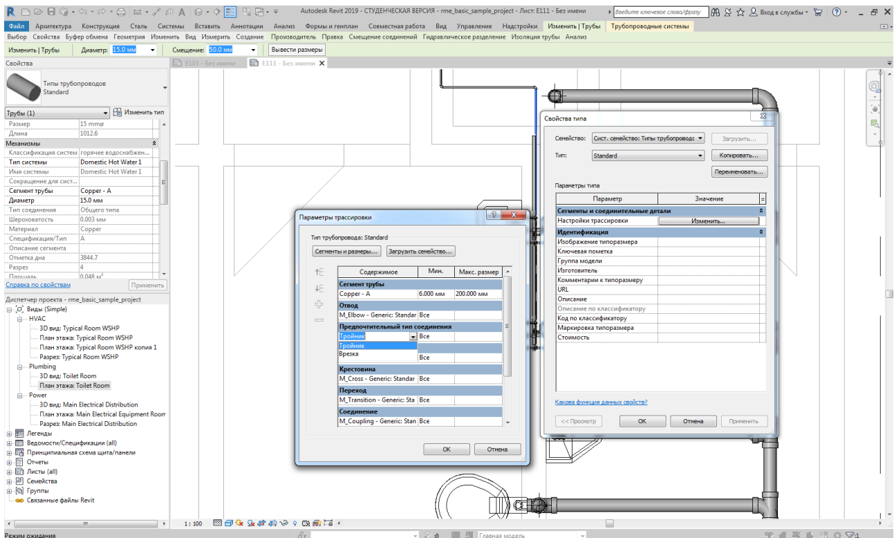
Рисунок 4.8. Задание типа соединения трубопровода
