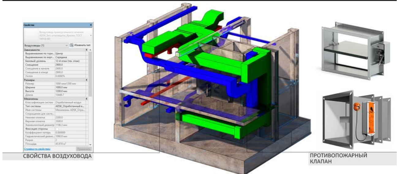
Рисунок 1.3. ВМ-проектирование приточных и вытяжных воздуховодов в здании
