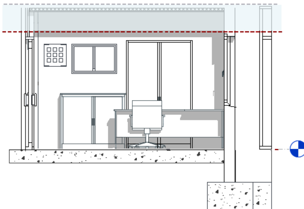
Рисунок 3.49. Секущий диапазон в плане потолка
