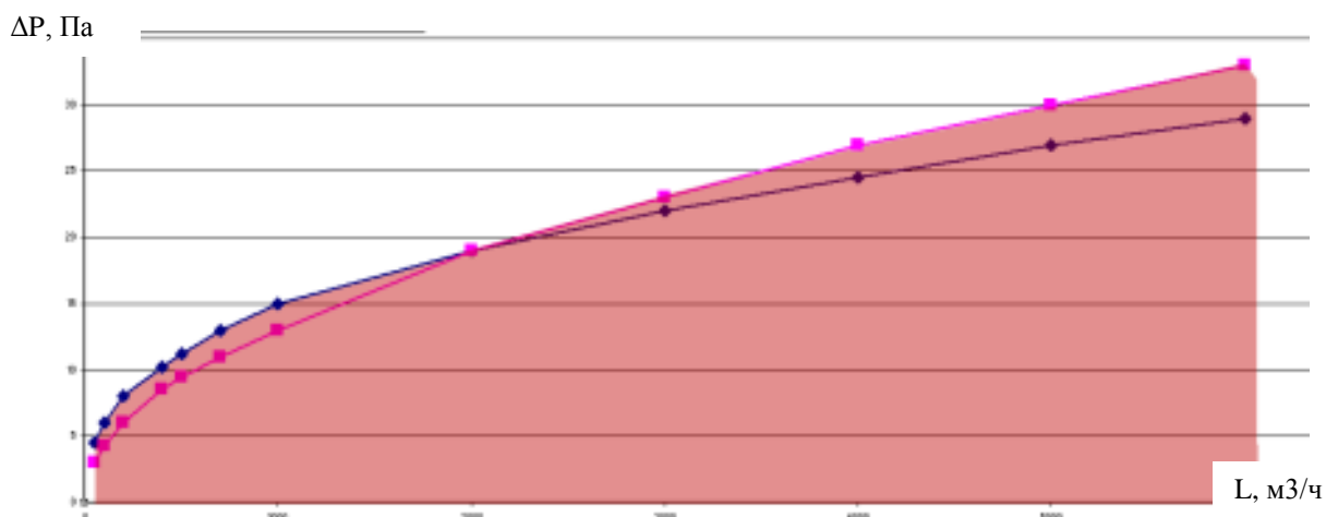
Рисунок 4.42. Определение размеров воздуховодов по трению (—●—) или скорости (—■—)
