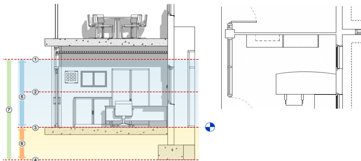
Рисунок 3.43. Фасад с указанием плоскостей секущего диапазона:
