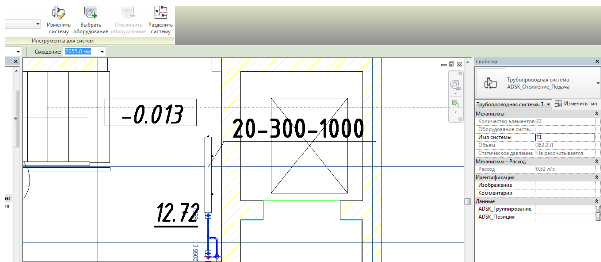
Рисунок 4.4. Задание имени системе трубопроводов
