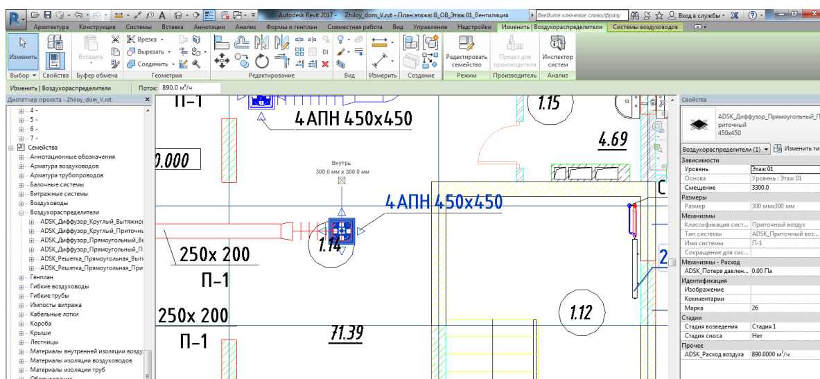
Рисунок 4.28. Расстановка воздухораспределителей и задание им расхода воздуха
