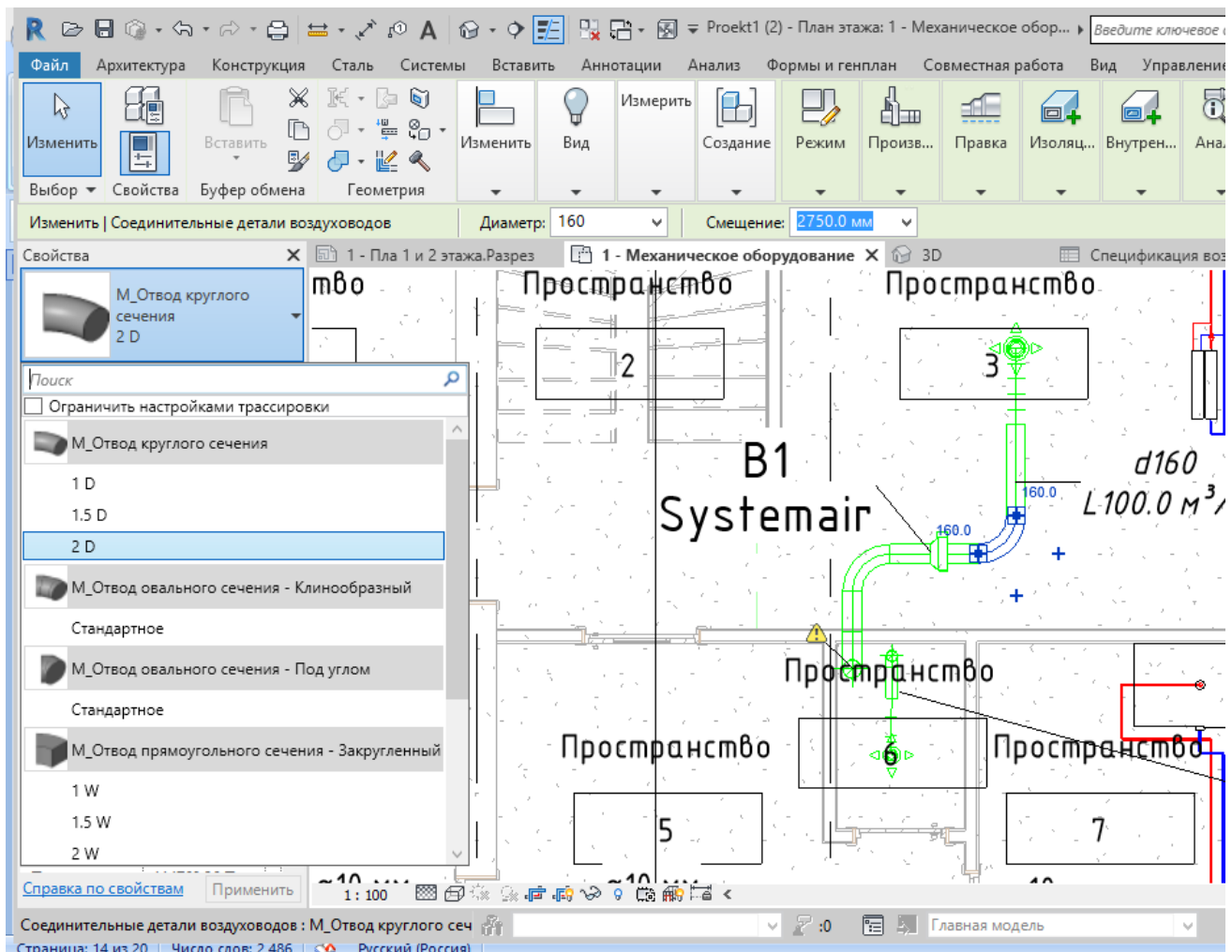
Рисунок 4.36. Изменение диаметра закругления
