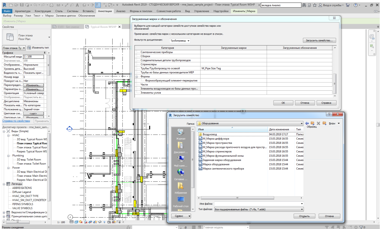
Рисунок 4.26. Окна Загруженные марки и обозначения и Загрузить семейство
