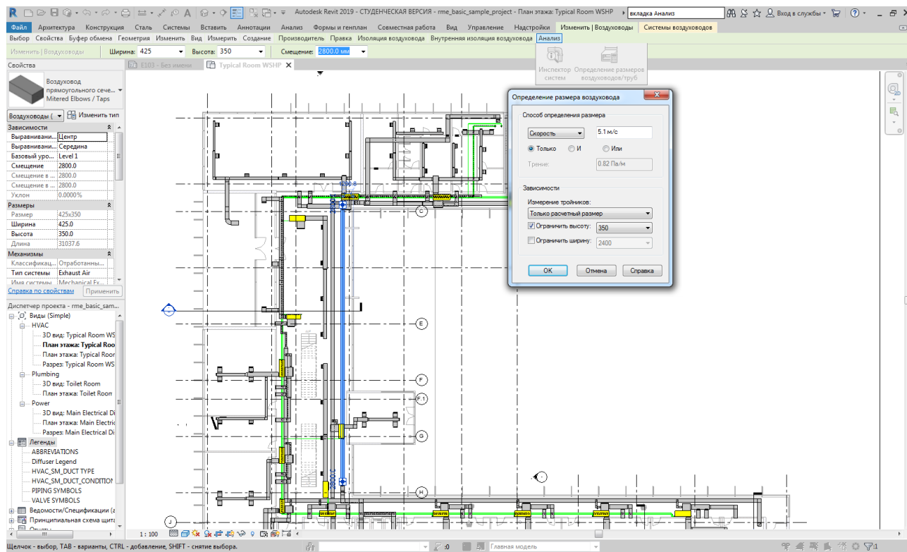
Рисунок 4.17. Ограничение высоты тройника
